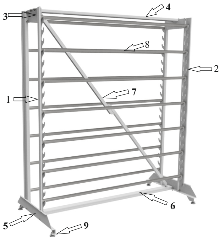
Состав комплекта стенда.
